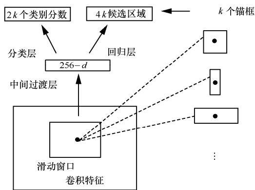
图3 区域提议网络结构 (RPN)
